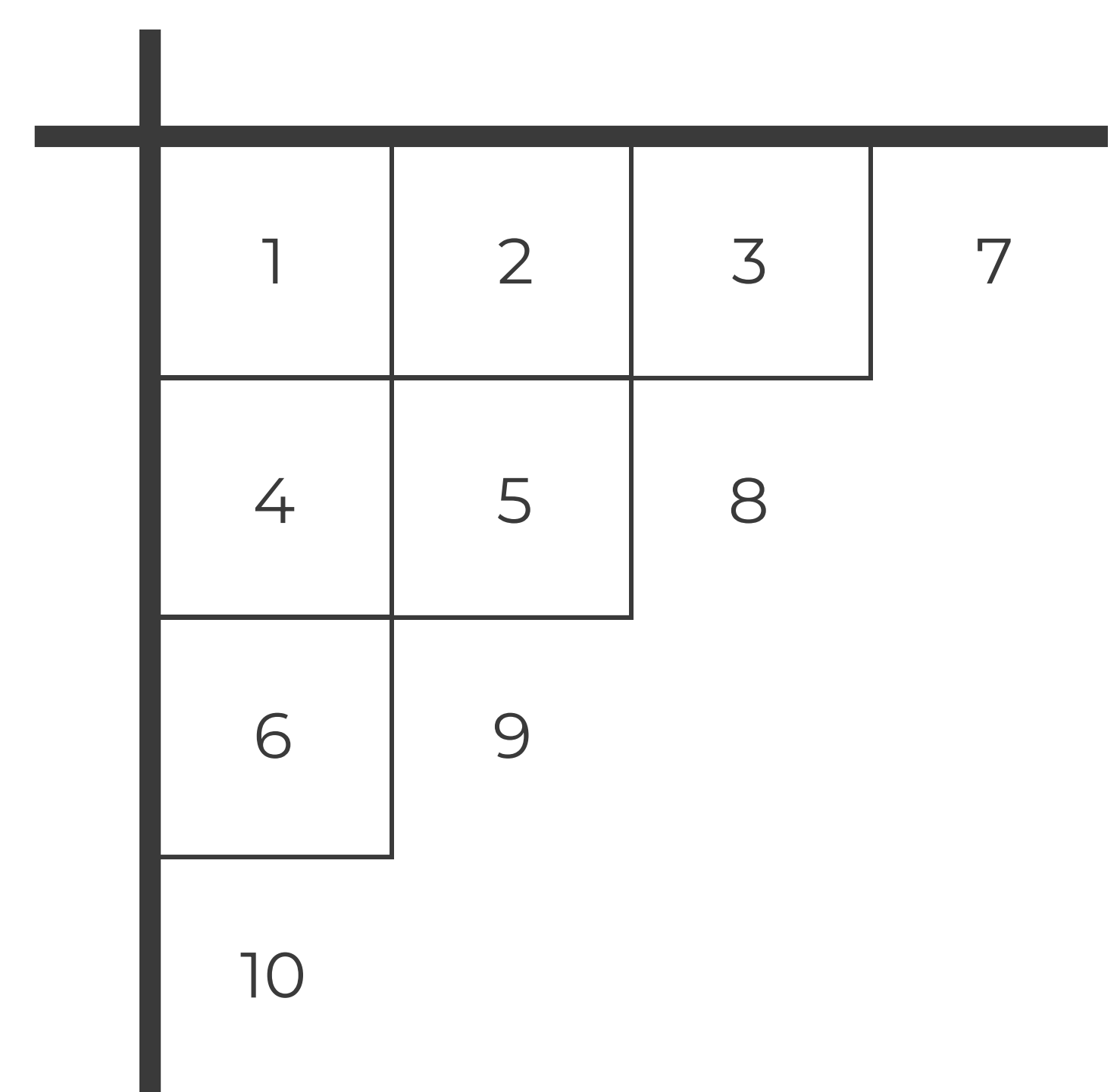
Рис. Порядок укладки плиток в квадрante
